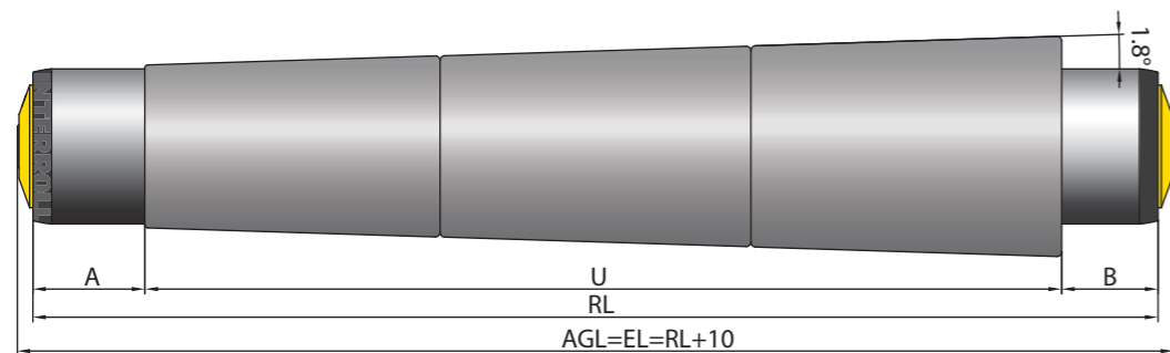
带 1.8° 内螺纹轴, 且右侧有管子突起的锥形元件
