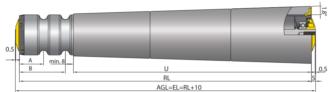
带 1.8° 内螺纹轴, 且右侧有管子突起的锥形元件
